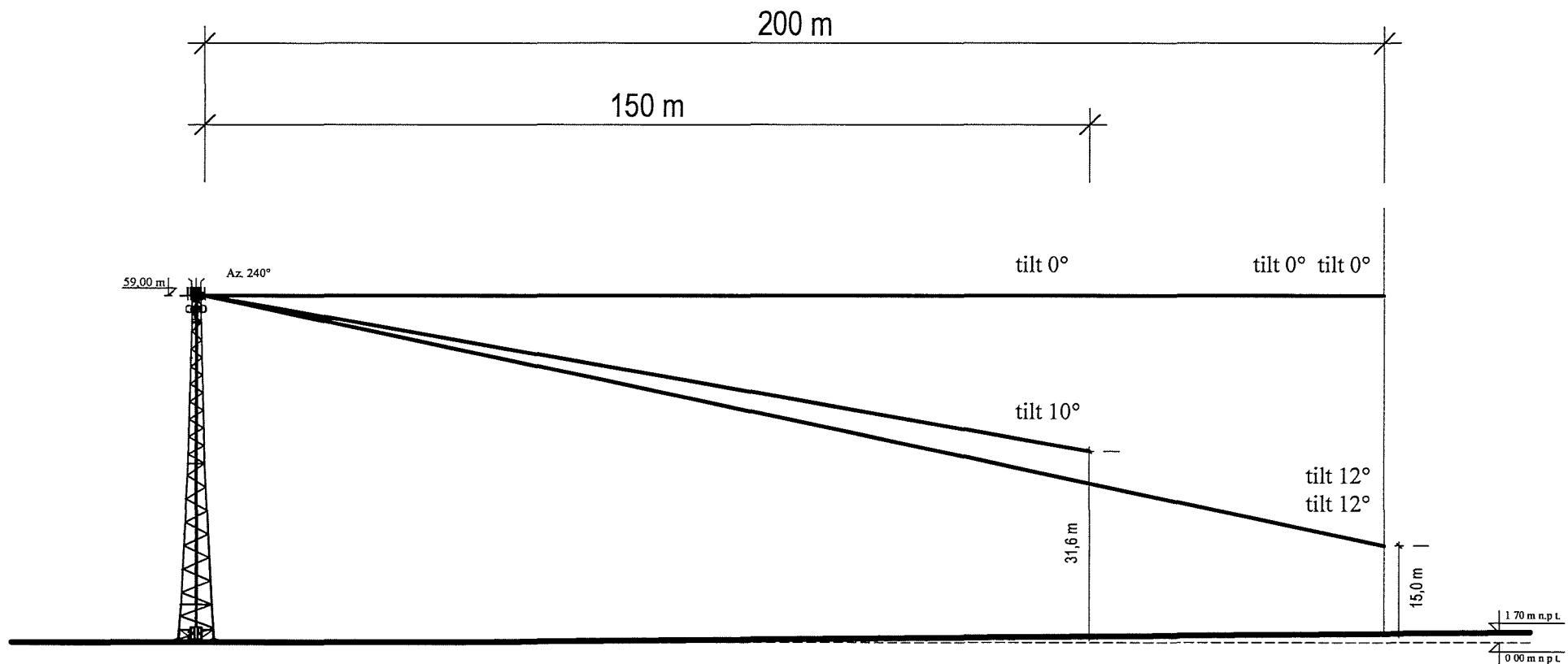
Rys. 4. Rzut pionowy osi głównej wiązki promieniowania na azymucie 240° w odległości do 150 i 200 metrów od środka elektrycznego anteny sektorowej dla tiltów 0°, 10° oraz 12°.
