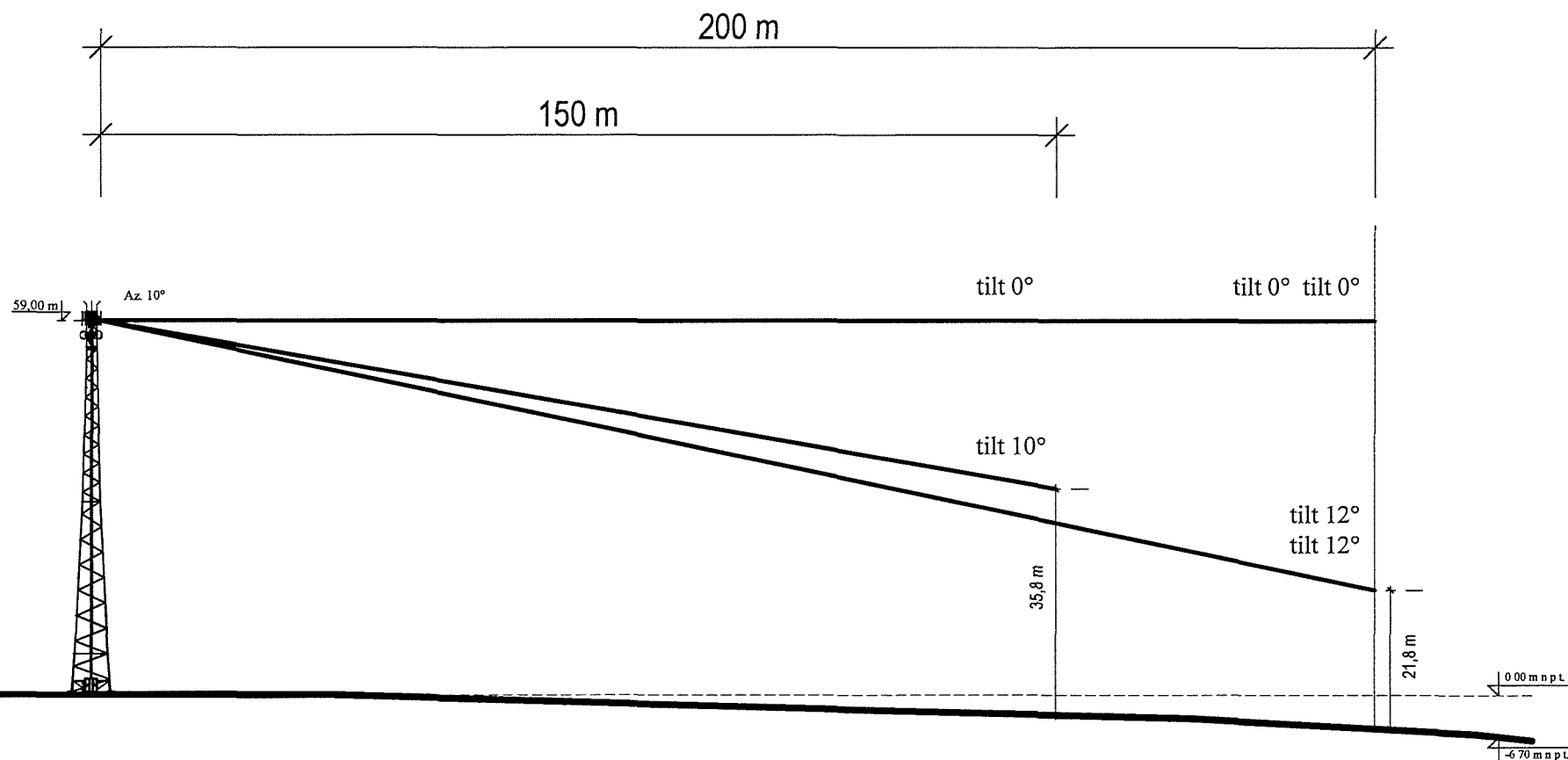
Rys. 2. Rzut pionowy osi głównej wiązki promieniowania na azymucie 10^\circ w odległości do 150 i 200 metrów od środka elektrycznego anteny sektorowej dla tiltów 0^\circ , 10^\circ oraz 12^\circ .
