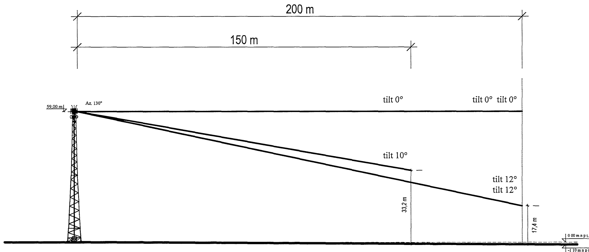
Rys. 3. Rzut pionowy osi głównej wiązki promieniowania na azymucie 130° w odległości do 150 i 200 metrów od środka elektrycznego anteny sektorowej dla tiltów 0°, 10° oraz 12°.
